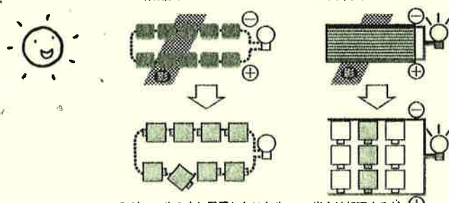
モジュールの中に発電しないセルがあると、回路全体が発電しない。
